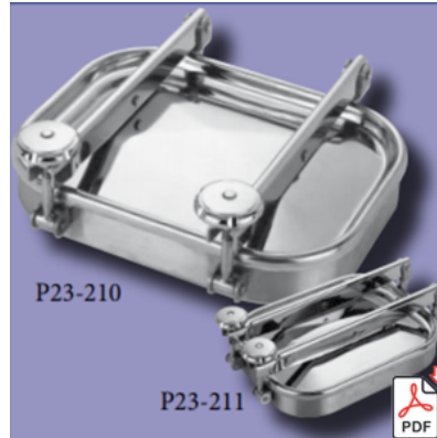
Cod. P3-P23-211 424x314 mm
