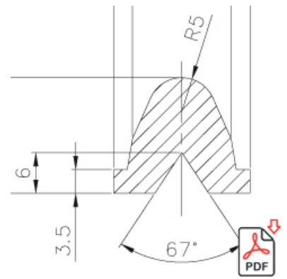
Těsnění
