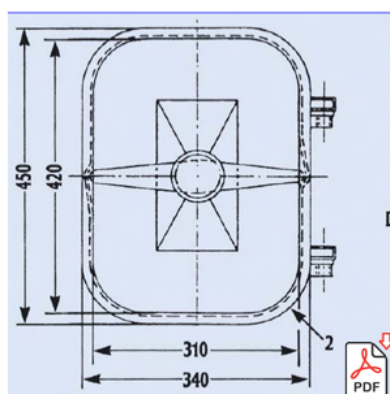
Cod. P3-P43-015 420 x 310 mm
