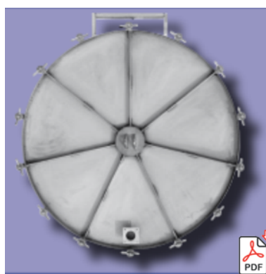
Cod. P22-1600 Ø 1600 mm 1 bar
